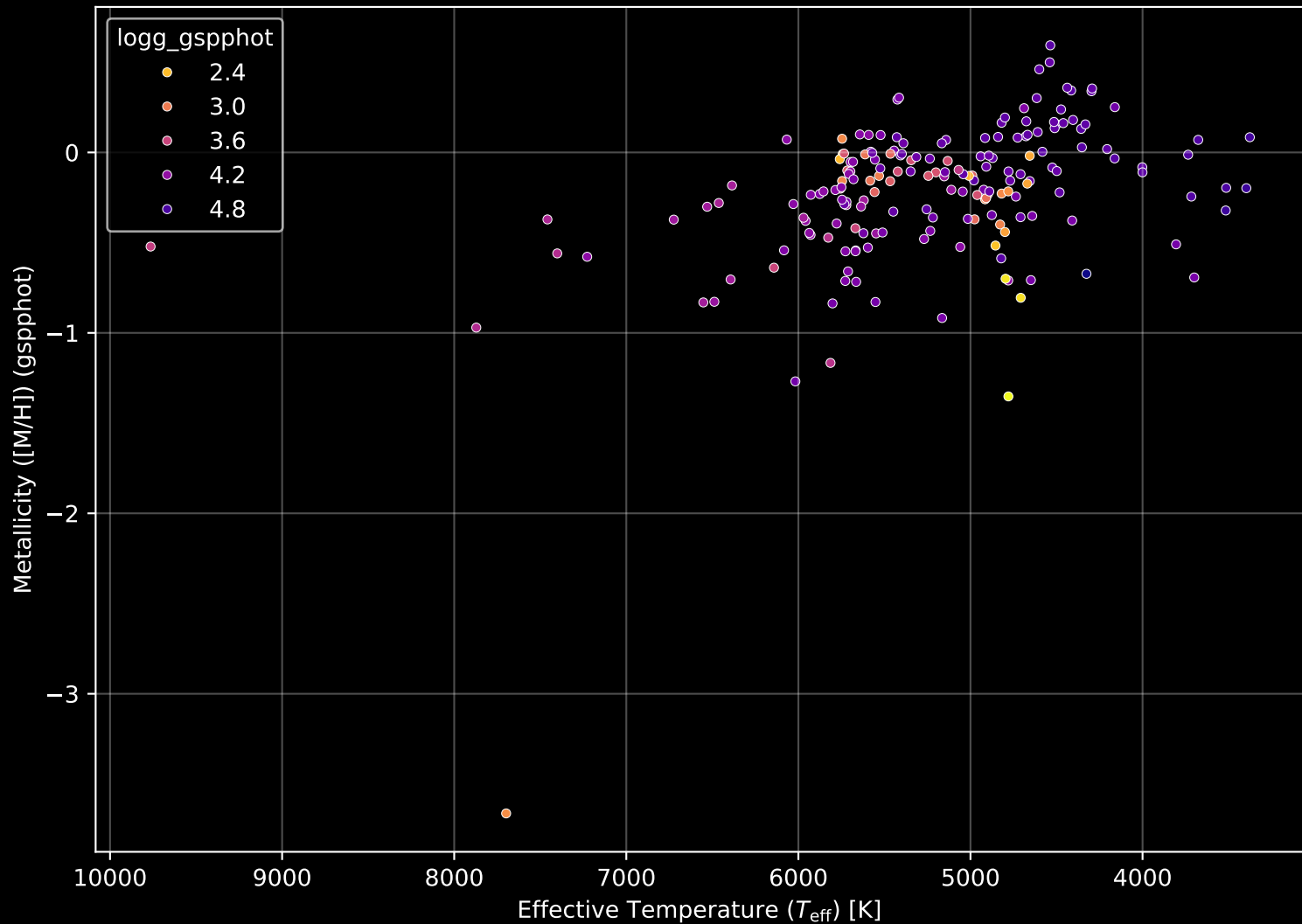
APOGEE DR17 Field: [042+68_btx] Stellar Population Parameters (n= 187)
